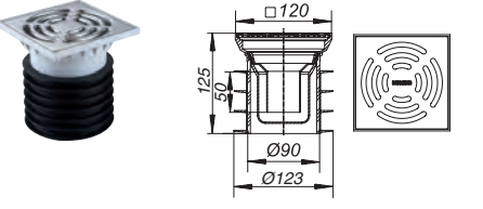
PRONTO K Ø 125 mm
