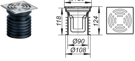
PRONTO Ø 110 mm
