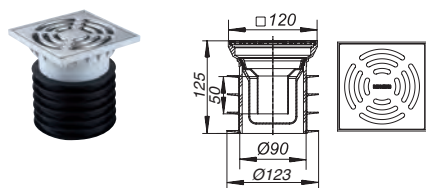
PRONTO K Ø 125 mm
