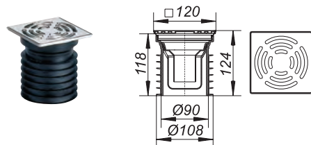
PRONTO Ø 110 mm
